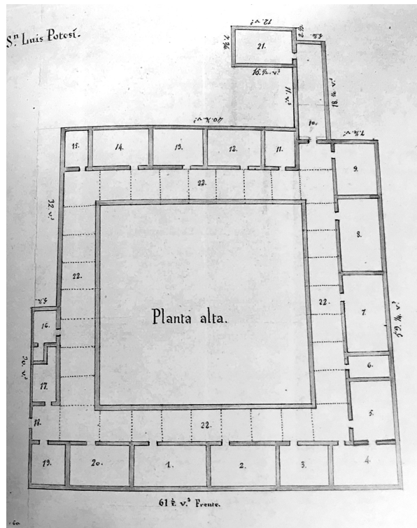
FIGURA 4. PLANTA ALTA DEL COLEGIO GUADALUPANO JOSEFINO
